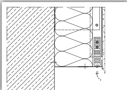
Aluminium Unterkonstruktion
