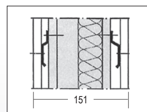
Basissystem CW 75/100 + RC 1 x 12,5 mm GK beidseitig R WR 46 dB, Prüfbericht Nr. 5
